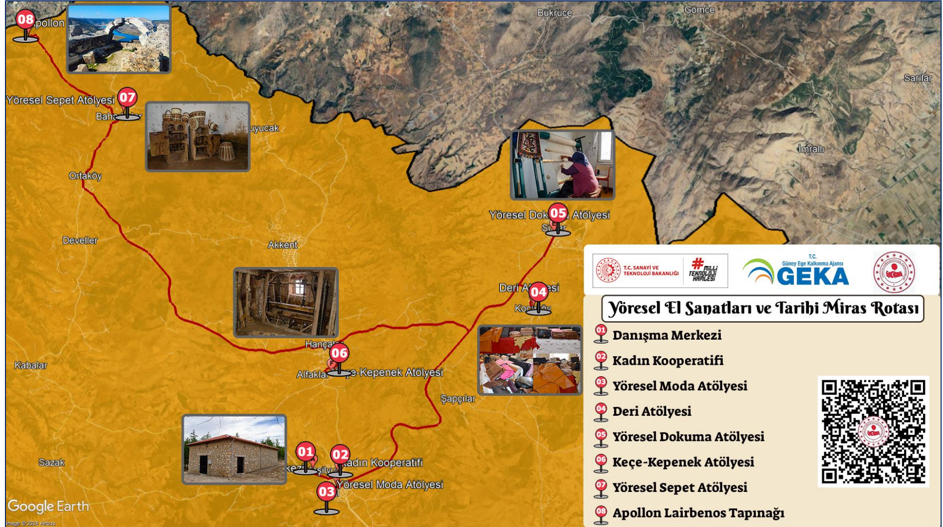
Şekil 26: Yöresel El Sanatları ve Tarihi Miras Rota Haritası
