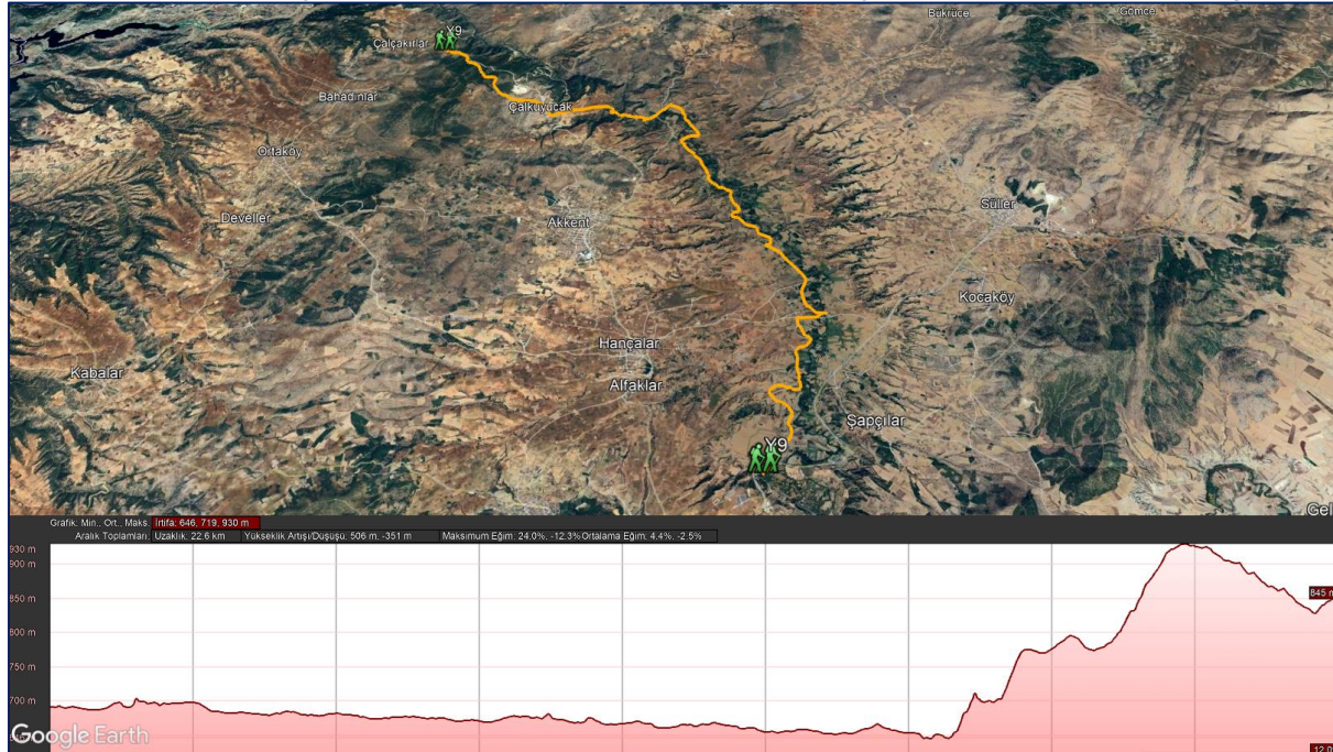
Şekil 40: Y9-Çakırlar Köyü-Menderes Yolu-Kumral Mesire Alanı Yürüyüş Rotası ve Yükseklik Grafiği
