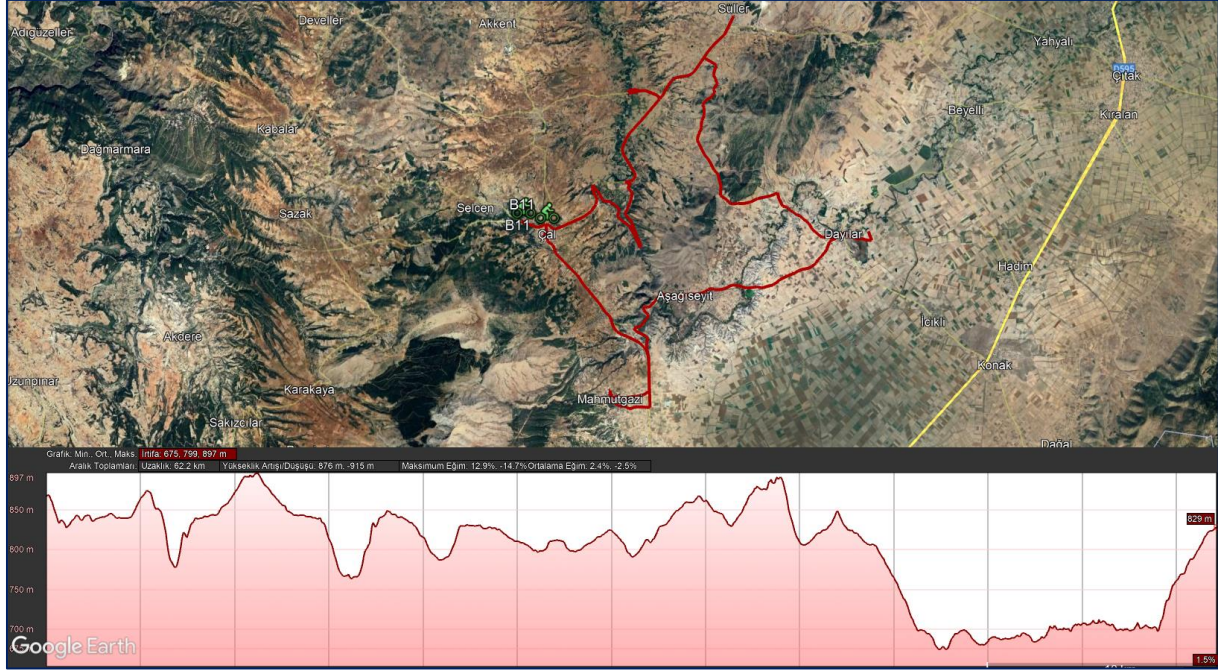
Şekil 55: B11-Danışma Merkezi-Kadın Kooperatifi Bisiklet Rotası ve Yükseklik Grafiği
