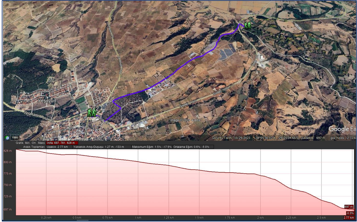
Şekil 31: Y2-Kadın Kooperatifi-Kumral Mesire Alanı Yürüyüş Rotası ve Yükseklik Grafiği
