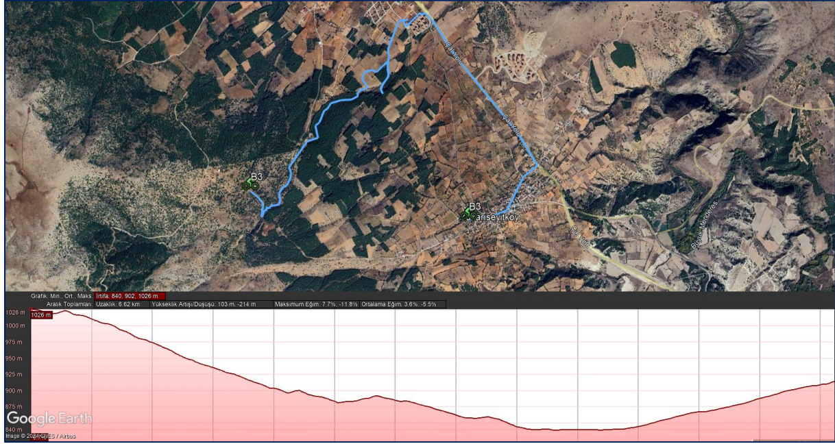
Şekil 47: B3-Yukarıseyit Bisiklet Rotası ve Yükseklik Grafiği
