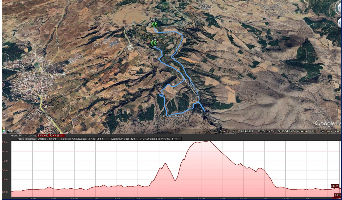
Şekil 35: Y5-Kısıc Kanyonu Yürüyüş Rotası ve Yükseklik Grafiği
