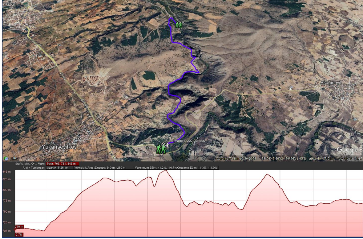
Şekil 33: Y4-Kısıc Kanyonu Yürüyüş Rotası ve Yükseklik Grafiği
