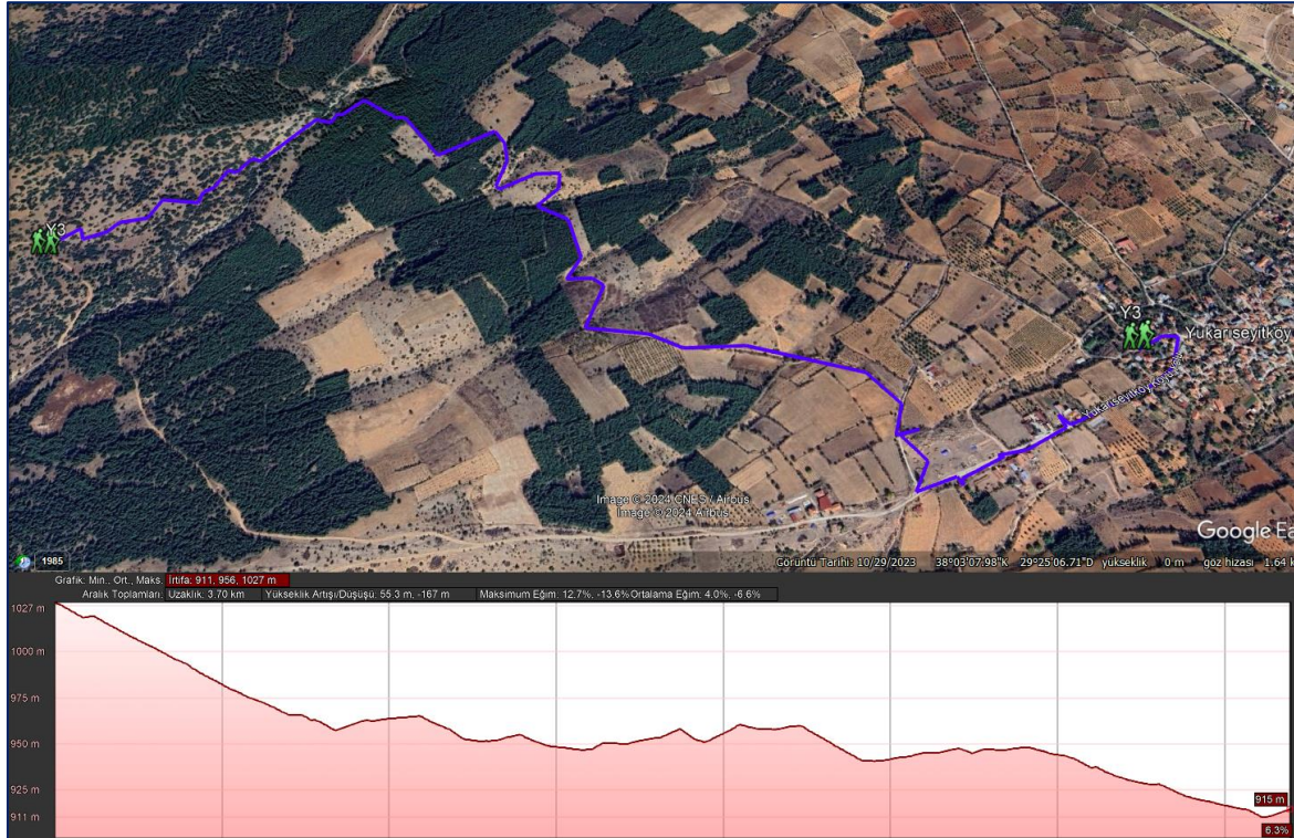
Şekil 32: Y3-Yukarıseyit Köyü Yürüyüş Rotası ve Yükseklik Grafiği
