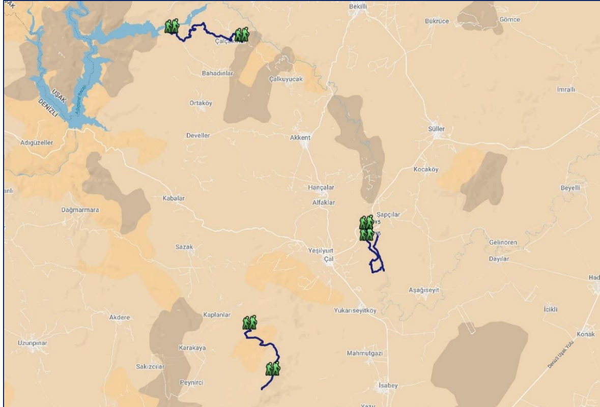
Şekil 34: 6-10 Kilometre Uzunluğundaki Rotalar
