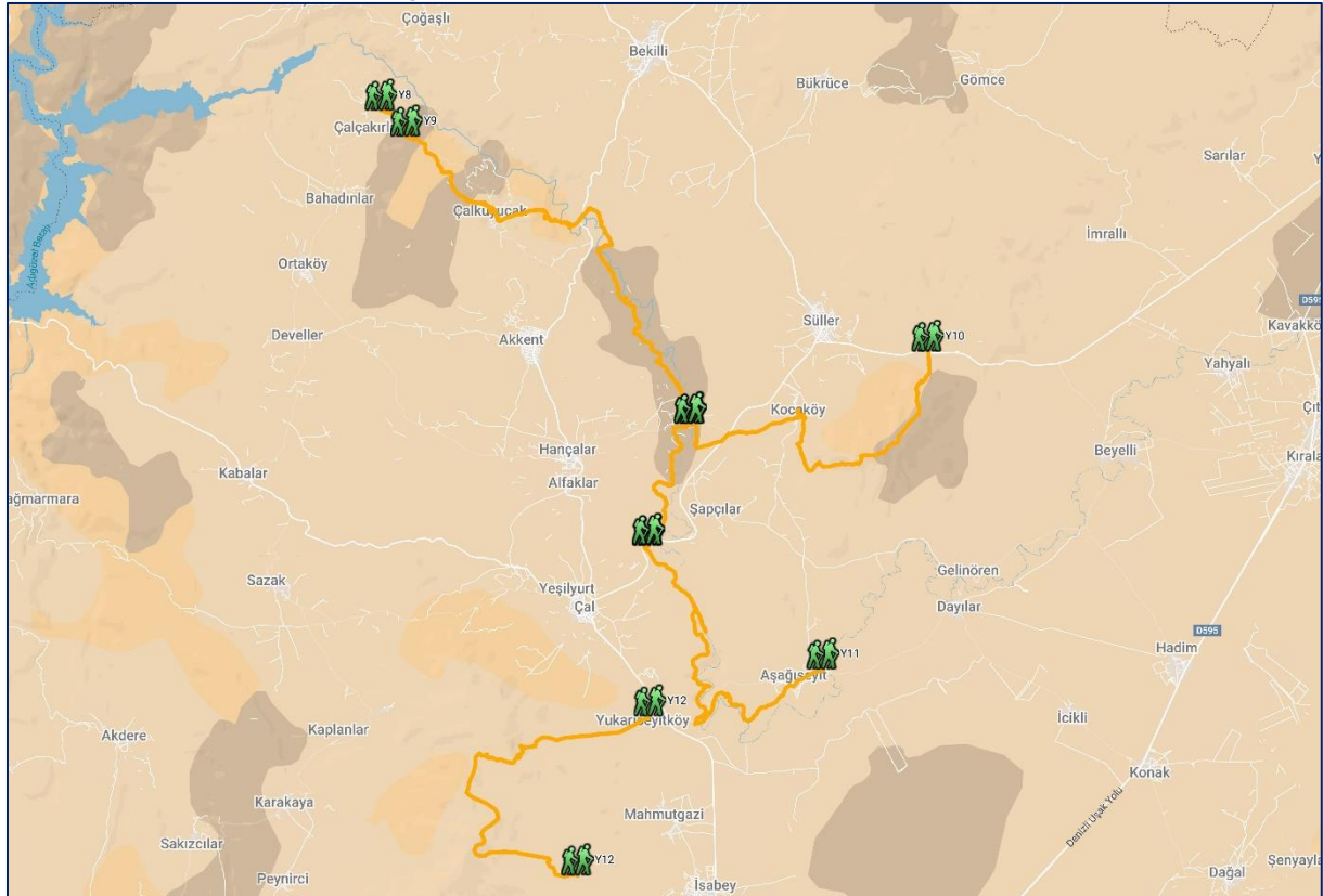
Şekil 38: 11-25 Kilometre Uzunluğundaki Rotalar
