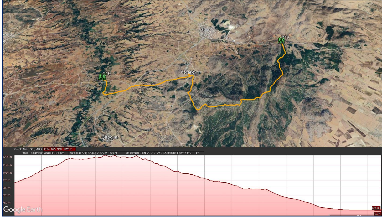
Şekil 41: Y10-Kocaköy Rotası Yürüyüş Rotası ve Yükseklik Grafiği
