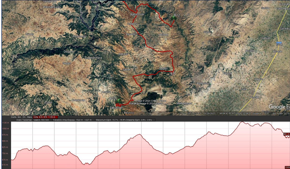
Şekil 56: B12-Menderes Vadi-Ağlayan Kaya Bisiklet Rotası ve Yükseklik Grafiği
