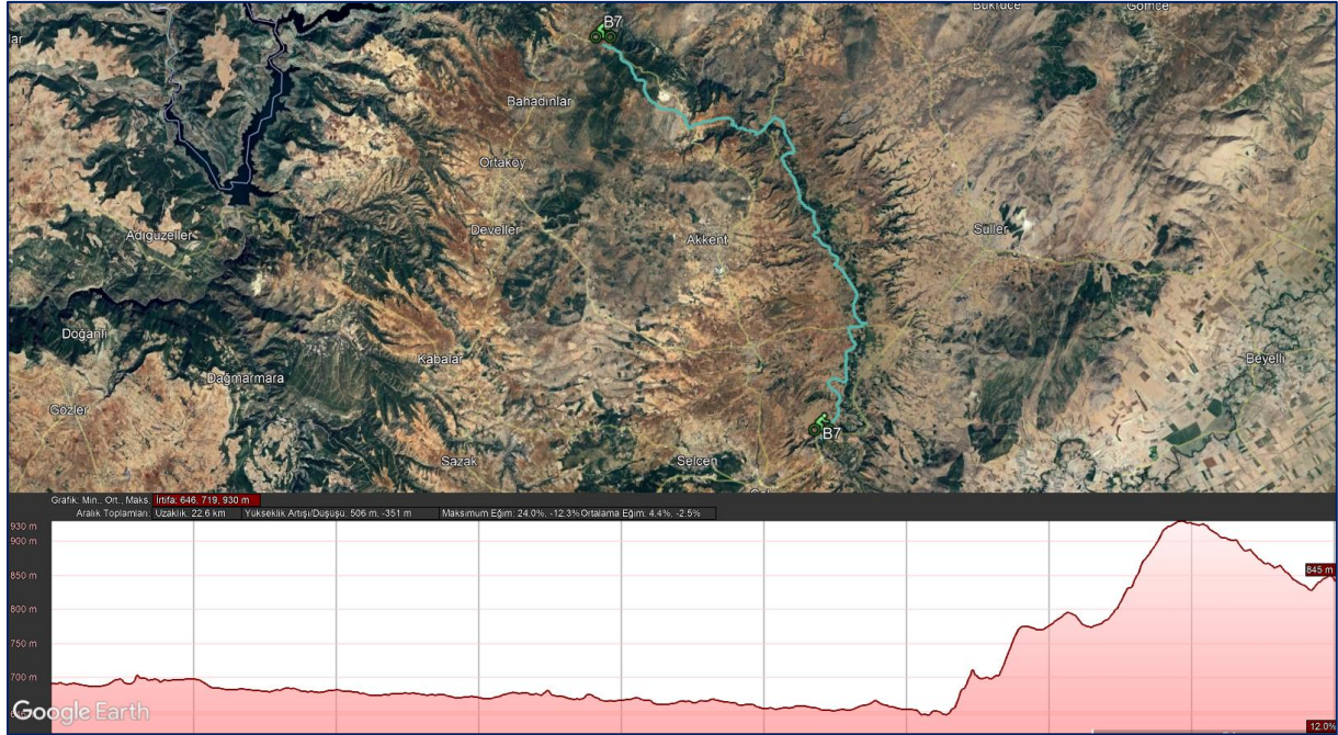
Şekil 51: B7-Çalçakırlar-Kumral-Menderes Yolu Bisiklet Rotası ve Yükseklik Grafiği
