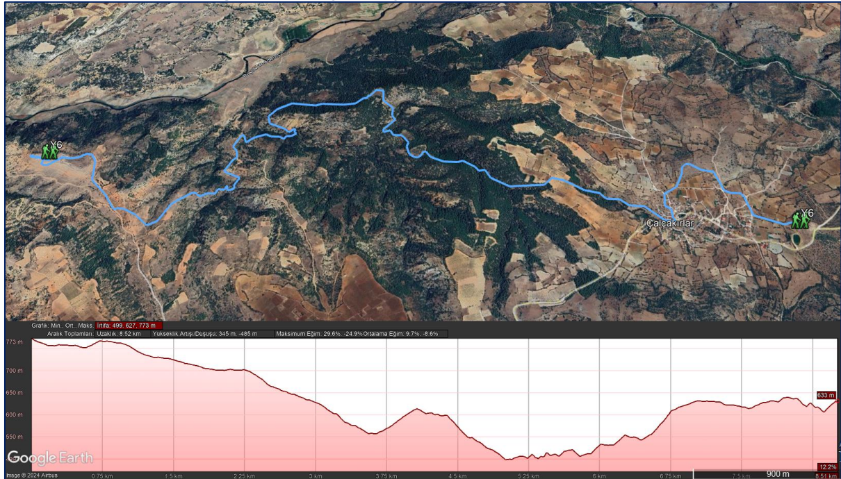
Şekil 36: Y6-Apollon Tapınağı-Çakırlar Köyü Yürüyüş Rotası ve Yükseklik Grafiği
