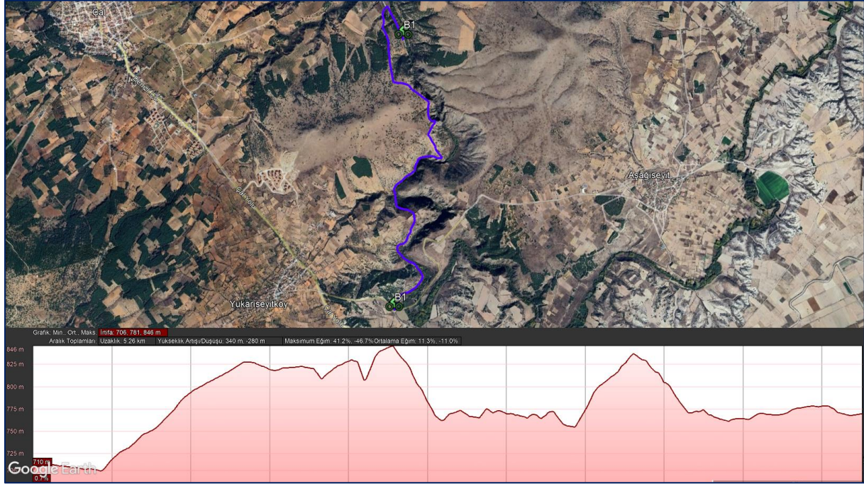
Şekil 45: B1-Kısıc Kanyonu Bisiklet Rotası ve Yükseklik Grafiği
