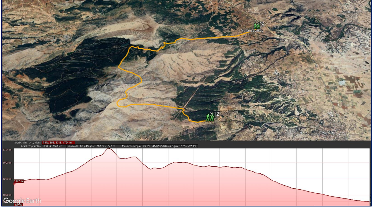
Şekil 43: Y12-İsabey-Çökelez Dağı-Yukarıseyit Yürüyüş Rotası ve Yükseklik Grafiği
