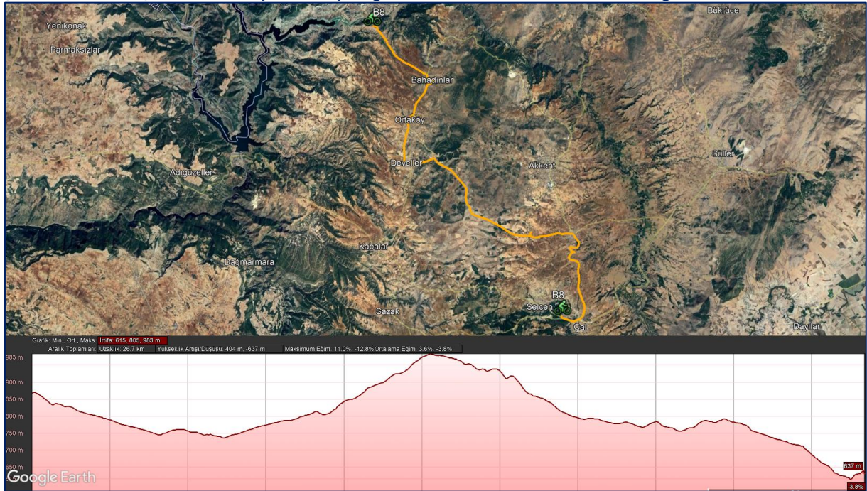
Şekil 52: B8-Danışma Merkezi-Apollon Tapınağı Bisiklet Rotası ve Yükseklik Grafiği
