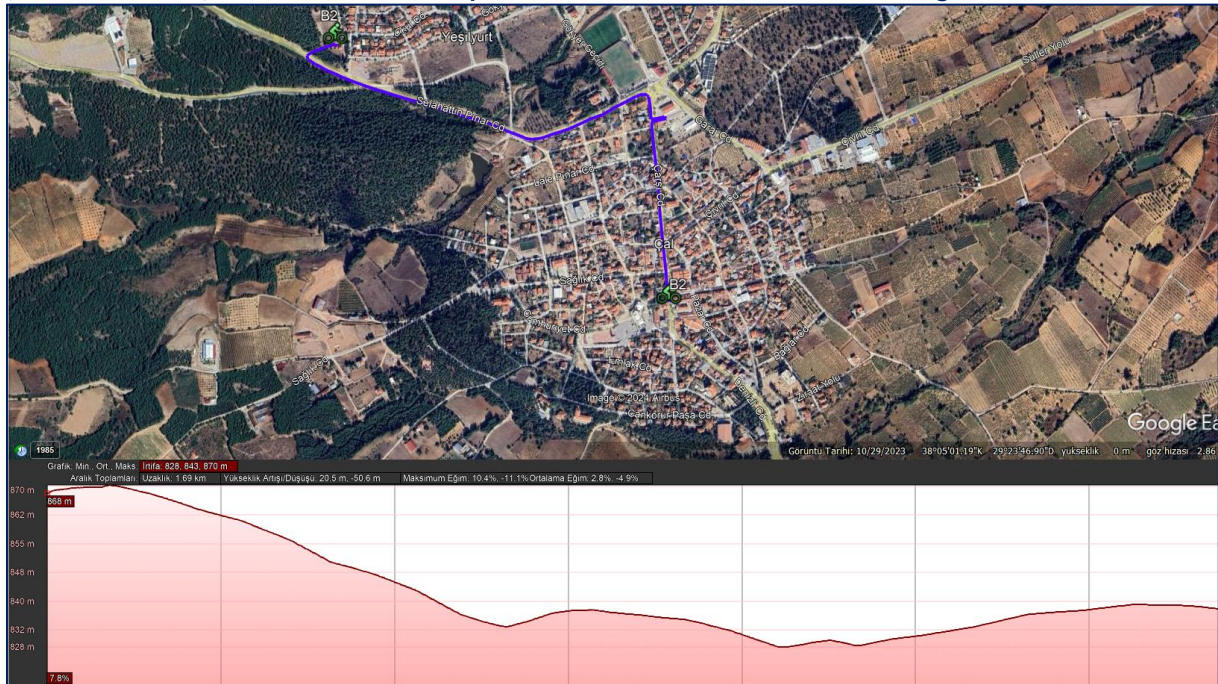
Şekil 46: B2-Danışma Merkezi-Kadın Kooperatifi Bisiklet Rotası ve Yükseklik Grafiği
