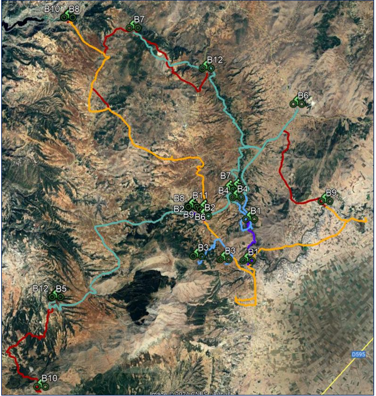
Şekil 44: Çal İlçesi Bisiklet Rotaları Haritası
