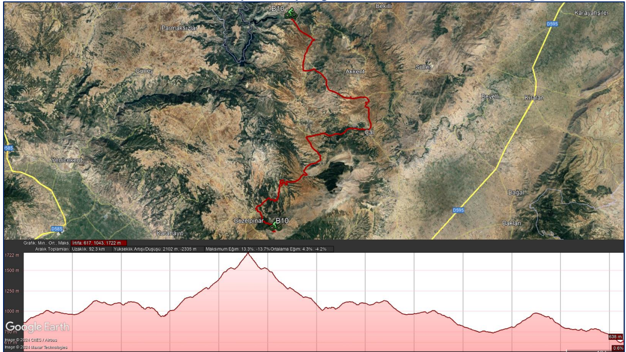
Şekil 54: B10-Çökelez Yamaç Paraşütü-Apollon Tapınağı Bisiklet Rotası ve Yükseklik Grafiği
